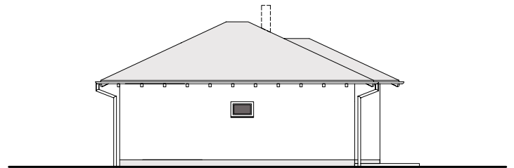
POHLED P4
