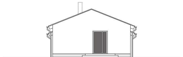
POHLED P4
